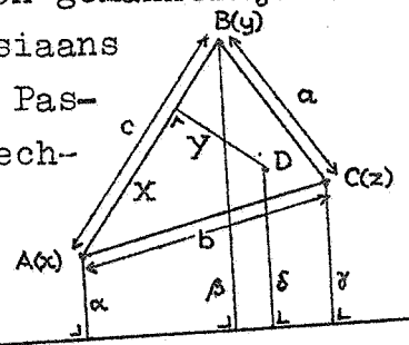
Fig. 3. Basisdriehoek in het metrische vlak.
