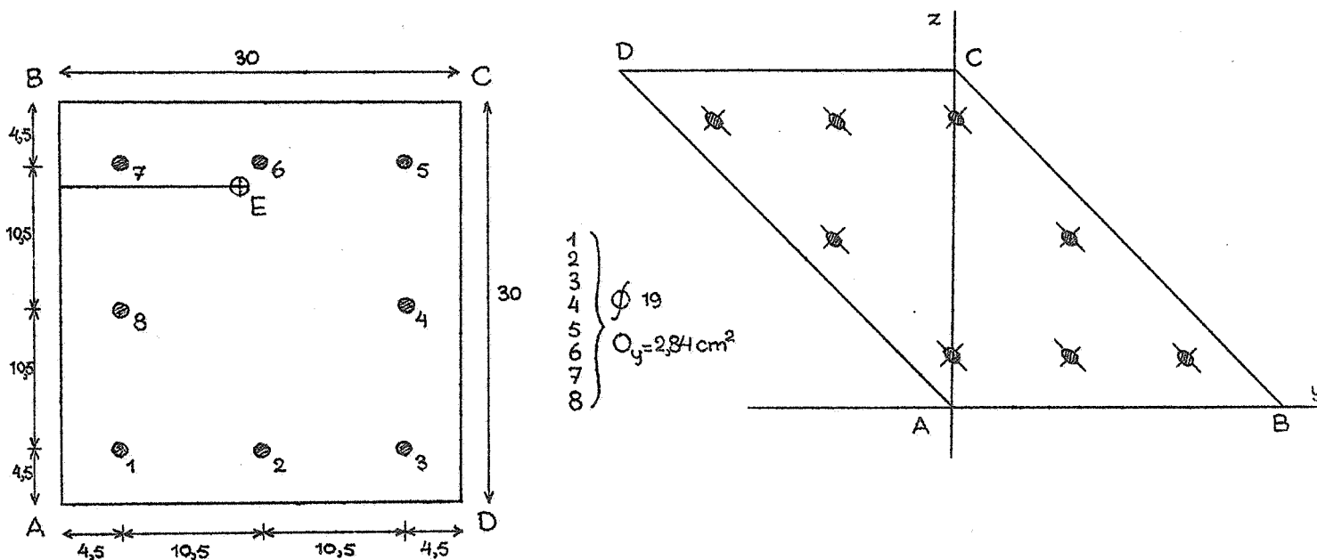
Fig.11. Betondoorsnede, metrisch en barycentrisch.
